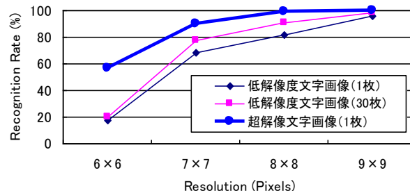
図 5. 撮影文字画像サイズと認識率の関係
