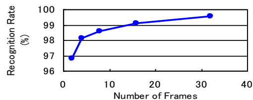
図 7. 用いる低解像度画像枚数と認識率の関係
