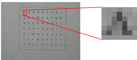
図 3. 実際に撮影された画像 ( 320 \times 240 pixels)
